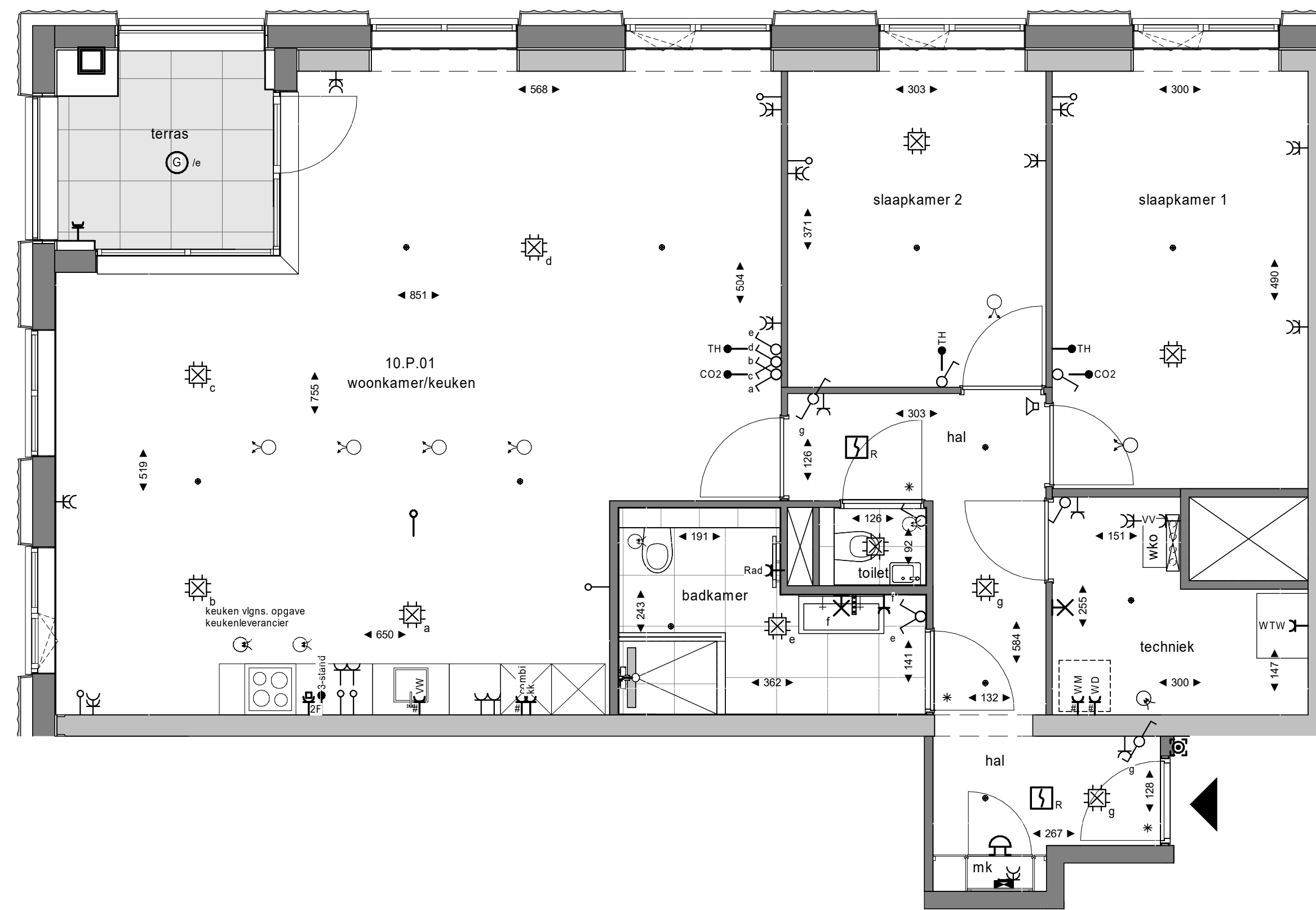
plattegrond 1 : 50 10e verdieping
